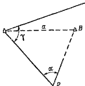
Рисунок А.2 – Схема комбинированной засечки
