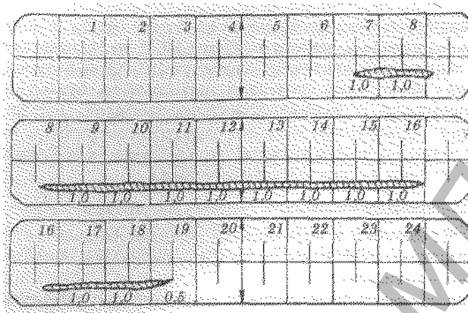
Рисунок 5 – Запись на ленте гелиографа в случае нарушения фокусного расстояния
