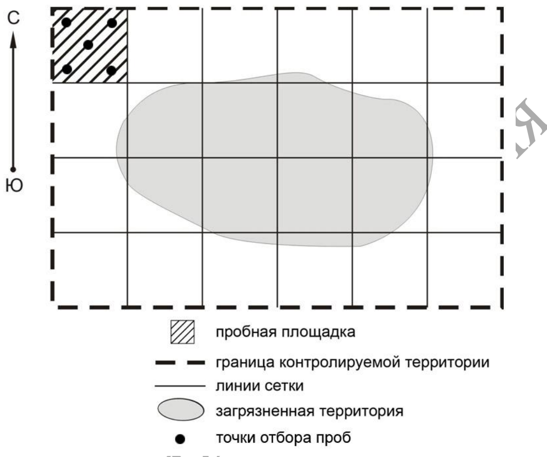
Рисунок А.1 – Расположение пробных площадок и точек отбора проб почв по систематической прямоугольной сетке
