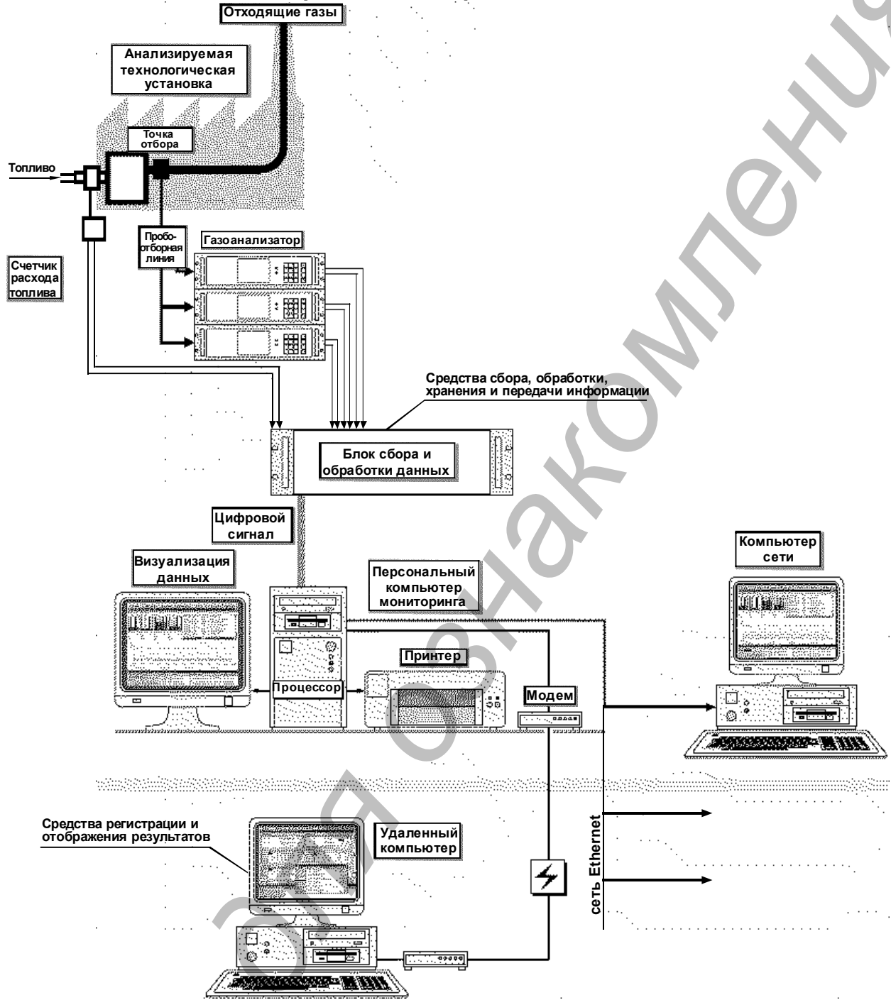
Рисунок А.2 – Основные узлы АСК и их взаимосвязь при определении расхода отходящих газов посредством измерения расхода топлива (для котельных установок)
