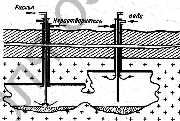
Рисунок 5 – Схема разработки «батаре́йным» методом (сдвоенная камера)
