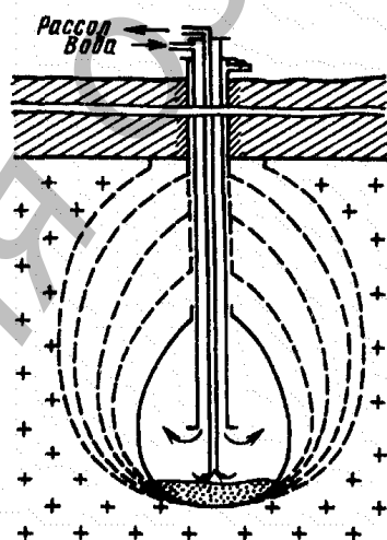
Рисунок 3 – Схема разработки с использованием метода «без нерастворителя»
