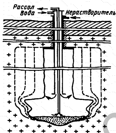
Рисунок 2 – Схема разработки с использованием метода «с заглубленной водоподачей»
